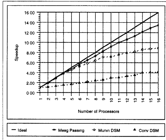
Fig. 10. Quicksort (QSORT).
